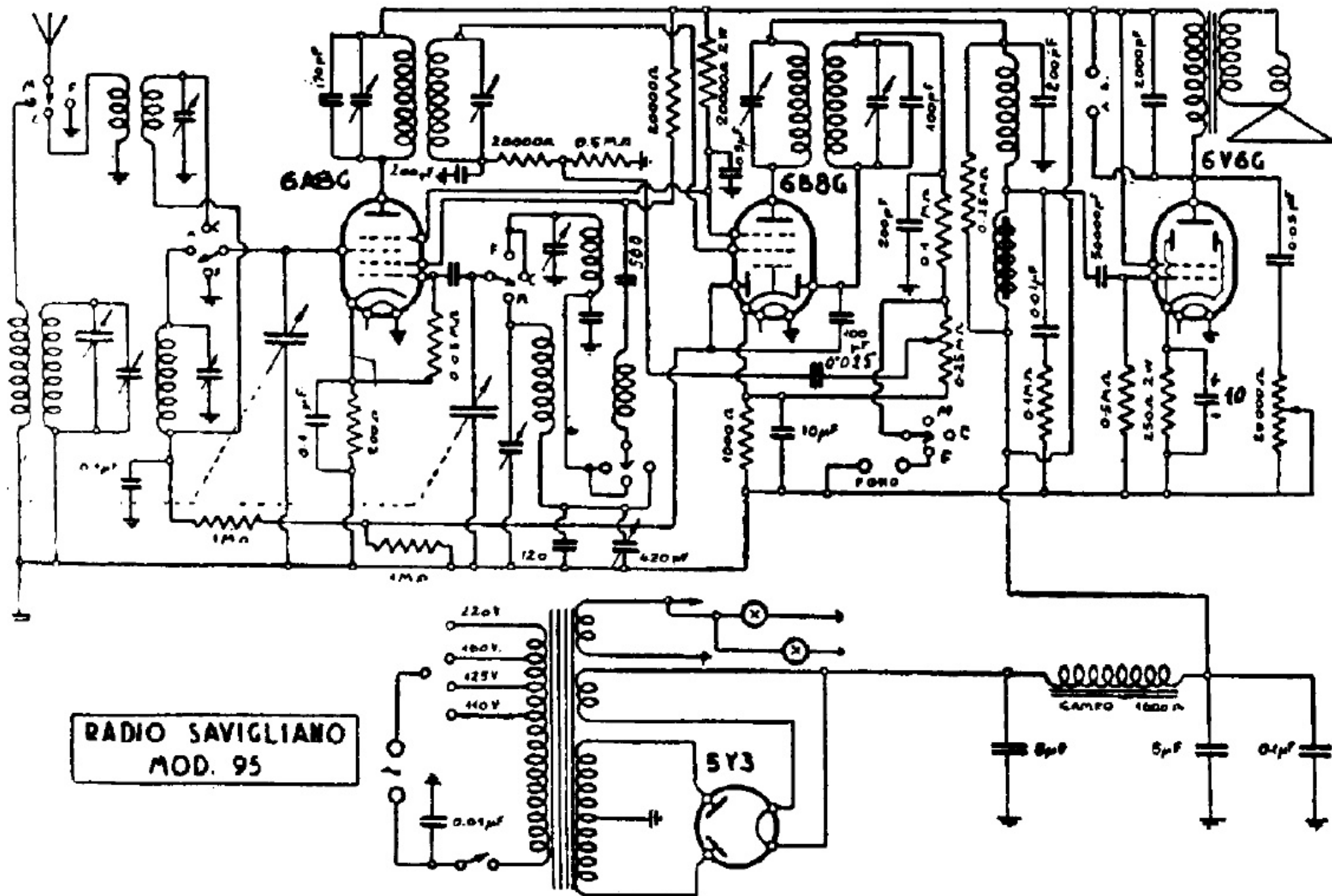
S. A. OFFICINE DI SAVIGLIANO — Mod 95 — Produzione 1938-39.
